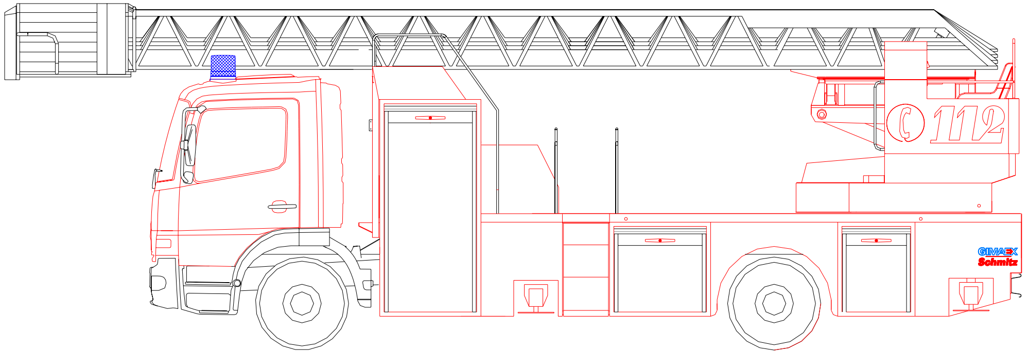
Drehleiter mit Korb DLA (K) 23/12
